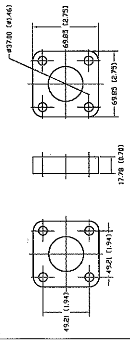
PE FOAM GASKET P/N 62950 1/4 SCALE
